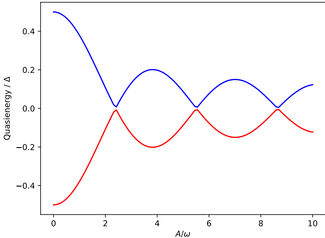
Floquet quasienergies
